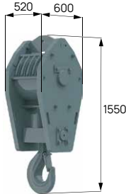
80t hook 单钩
