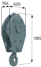
25t hook 单钩
